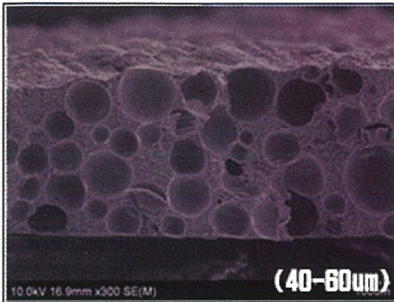
オプティマス断面図
